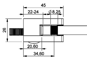
GERADER ANSCHLUSS
